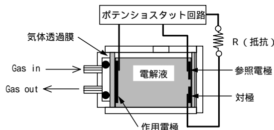
構造図
